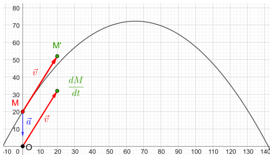
Position du point M(x, y) sur sa trajectoire y en fonction de x (en m ).
