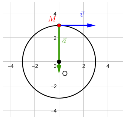
Figure - Trajectoire du point M : y en fonction de x . \vec{v}(0) et \vec{a}(0) . Voir animation.
